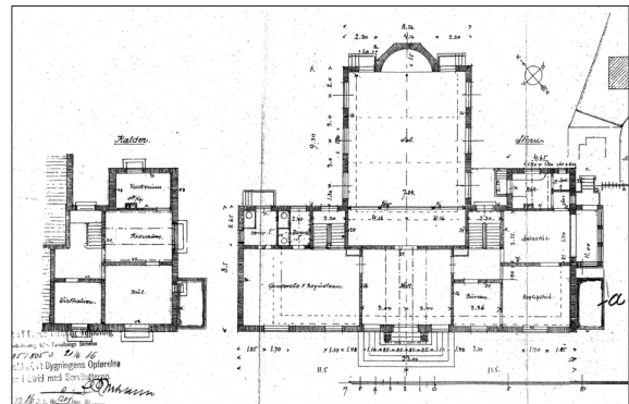
6.19 - Tegning af husets grundplan udfærdiget i 1916. Sådan var udformningen da Martinus købte huset. Det store rum opad på tegningen er det rum som Martinus indrettede til foredragssal, og som oprindeligt var udformet så det lignede et kirkerum. Den ene lejlighed er til højre for indgangen og den anden er på 1. sal. Kælderen ses til venstre på tegningen, den var, som vi kan se ikke så stor. Den blev senere udvidet i forbindelse med en større ombygning. - mi
